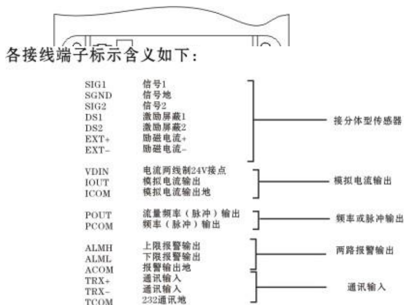
圆表端子接线与标示
