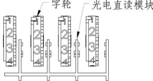
字轮与模块装配示意图
